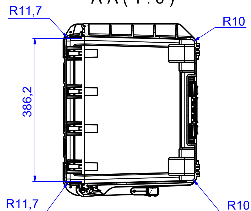
A-A ( 1 : 6 )
