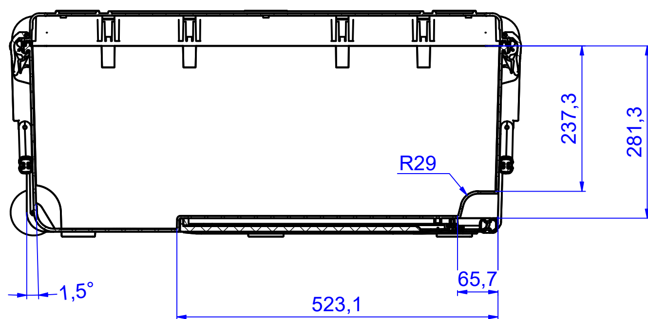
B-B ( 1 : 6 )
