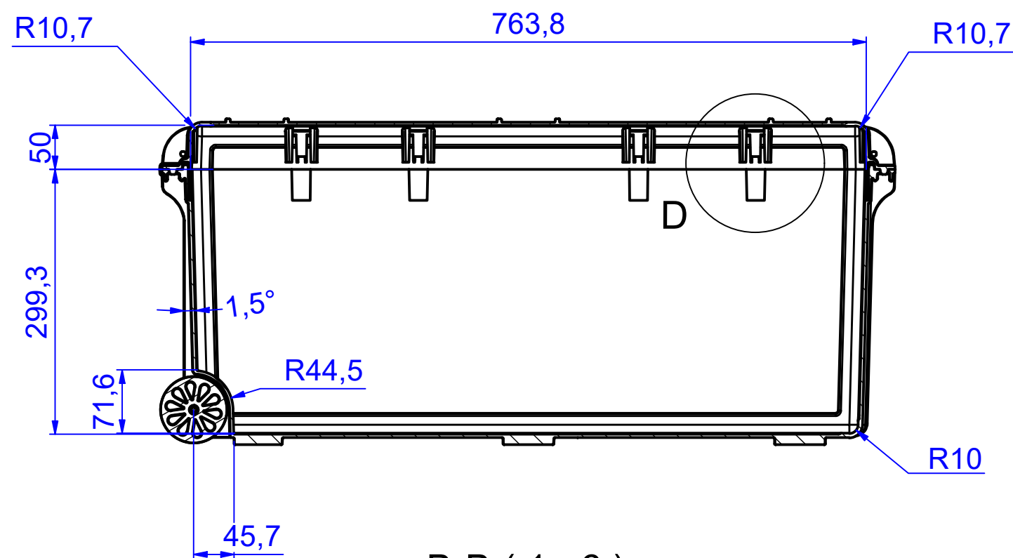
B-B ( 1 : 6 )
